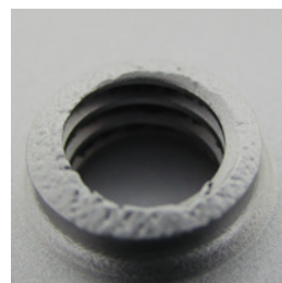
Filettatura foro con sbavatura
