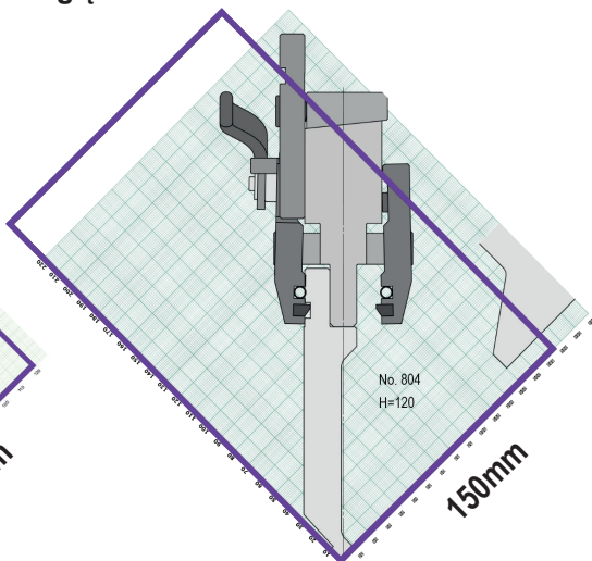
Nowe narzędzie AFH (H=120mm)
